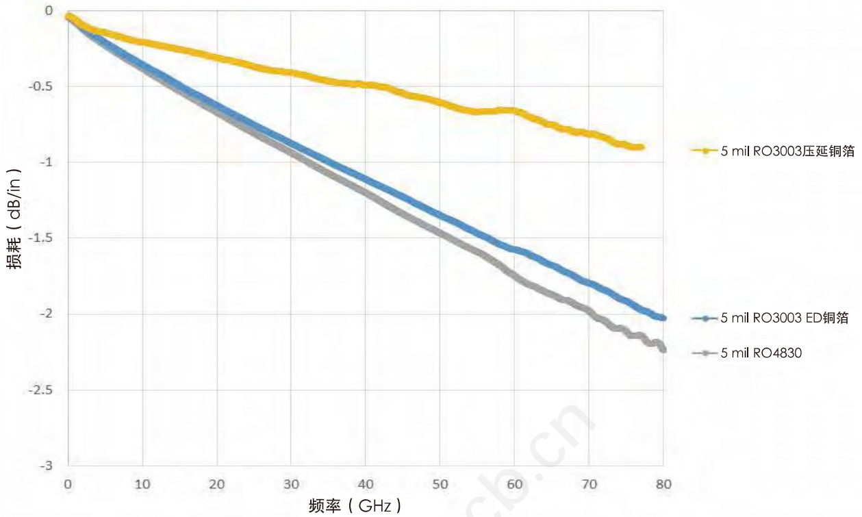
微带线插入损耗，差分长度方法 5 mil、9.4 mil RO4830™与5 mil RO3003™材料的比较
